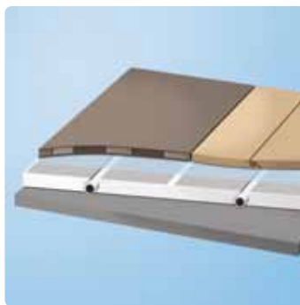
«Сухой» теплый пол, установленный на существующий пол
