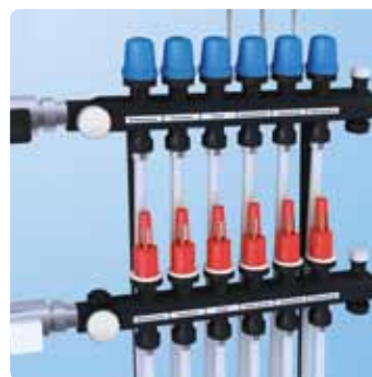
Пластиковый коллектор Uronor
